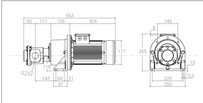
FOM 570- FOM 590 ( 2,2 kW ) weight: 41 kg
